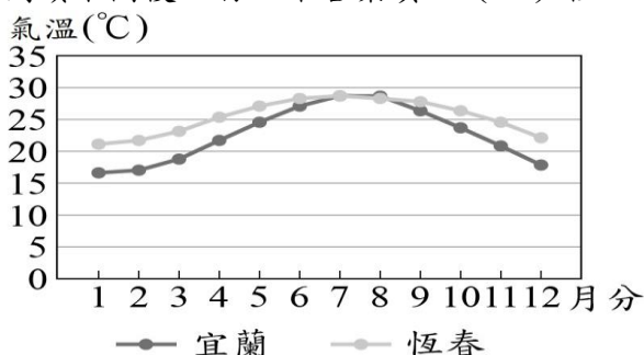
▲宜蘭、恆春月平均氣溫統計圖
